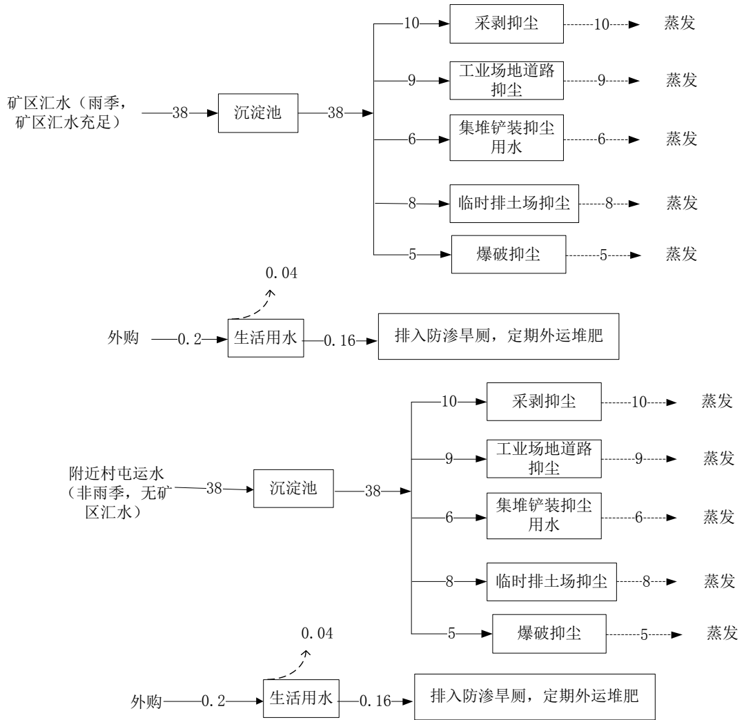
图 3-1-2 水平衡图 单位: m 3 /d
