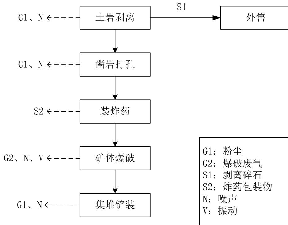
图 3-3-1 本项目开采工艺流程及产污环节示意图
